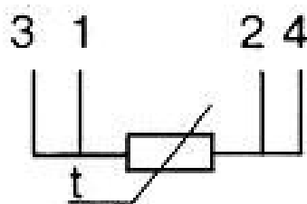
Рисунок А.1 – Четырехпроводная схема «4»
