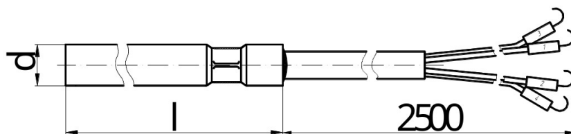
Рисунок Б.1 – ТСМ-0196-13...-20
