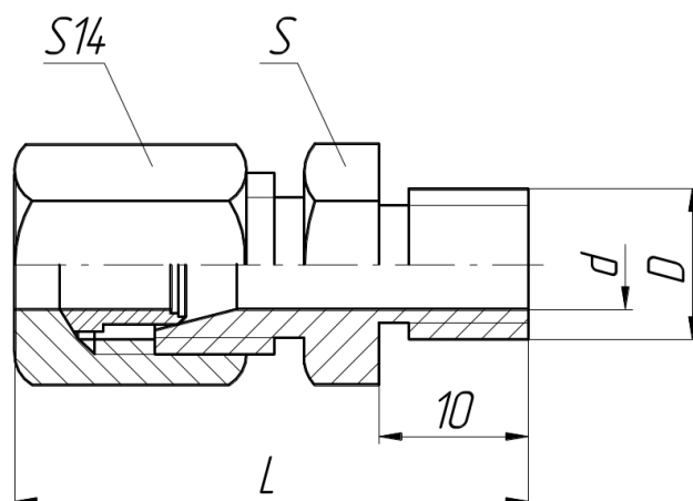
Рисунок В.1 – Штуцер 6.454.015
