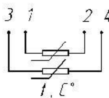
Рисунок А.2 – Схема «2х2»
