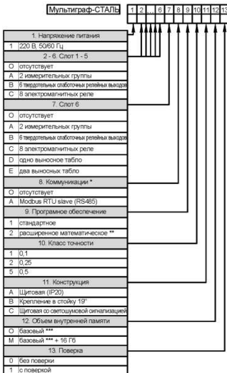
Схема заказа приборов Мультиграф-СТАЛЬ Карта заказа
