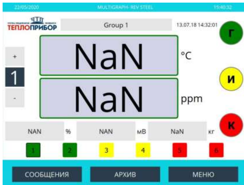
Рисунок 2.18 – Главное меню
