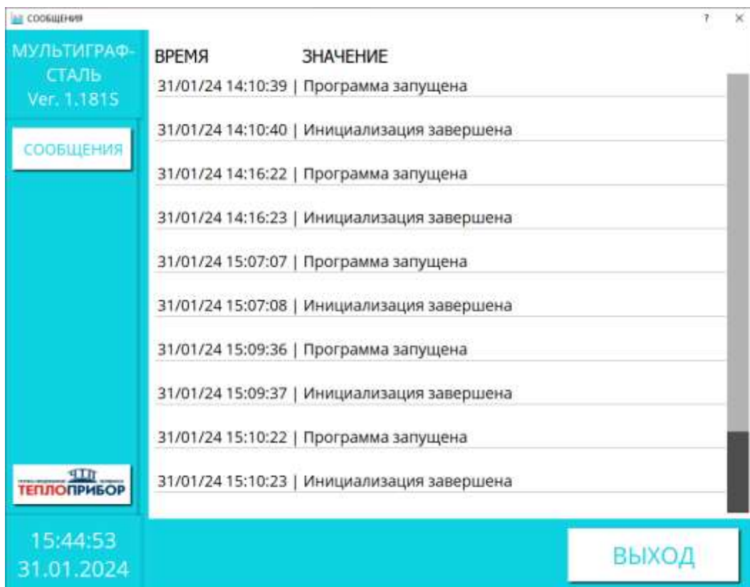
Рисунок 2.19 – Сообщения
